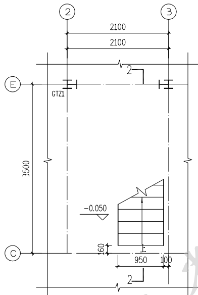
楼梯一层平面图 本楼梯适用于200平方米户型
