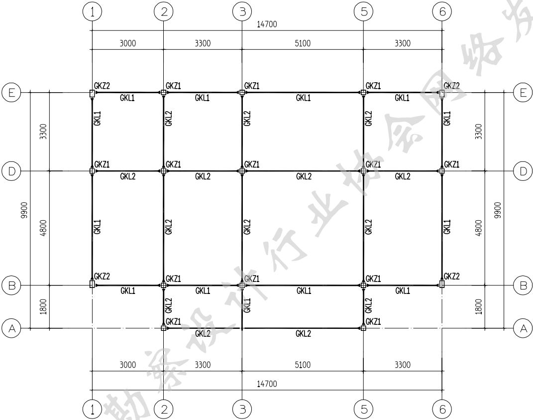
屋面结构平面布置图 6.130
