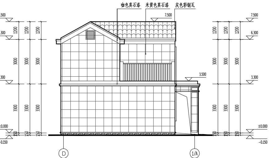
西立面图 1:100
