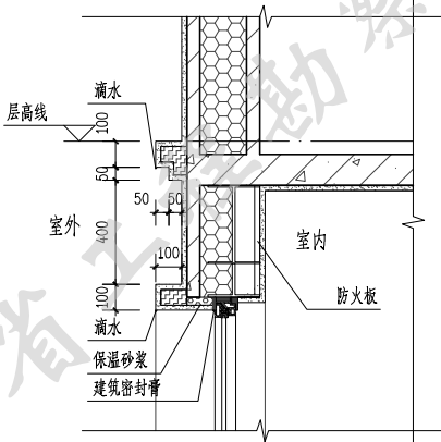
外窗上口节点、层间造型节点 1:20
