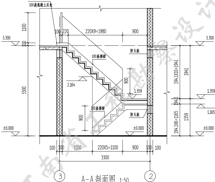
A-A剖面图 1:50
