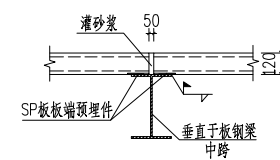
板与中间梁搭接做法
