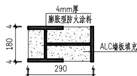
钢柱防火构造
