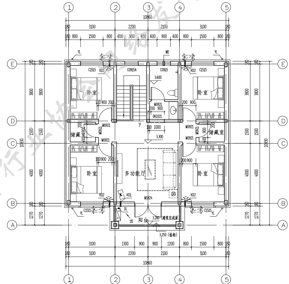
220平方米户型二层平面图 1:100
