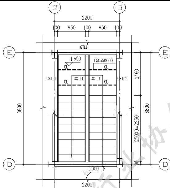
楼梯二层平面图
