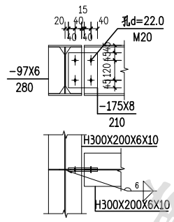
梁与梁铰接节点一
