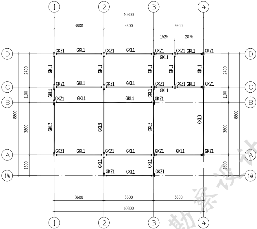
二層結構平面布置圖 3.130
