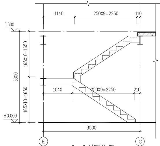
2-2剖面详图 本楼梯适用于200平方米户型
