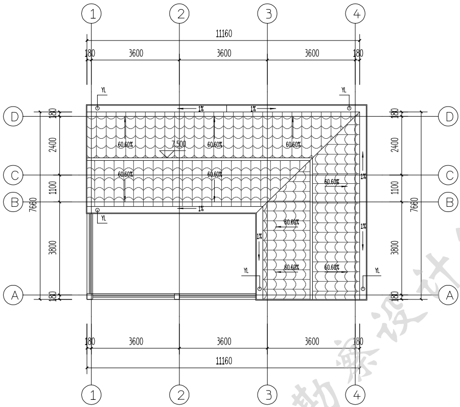
150平方米户型屋面层平面图 1:100
