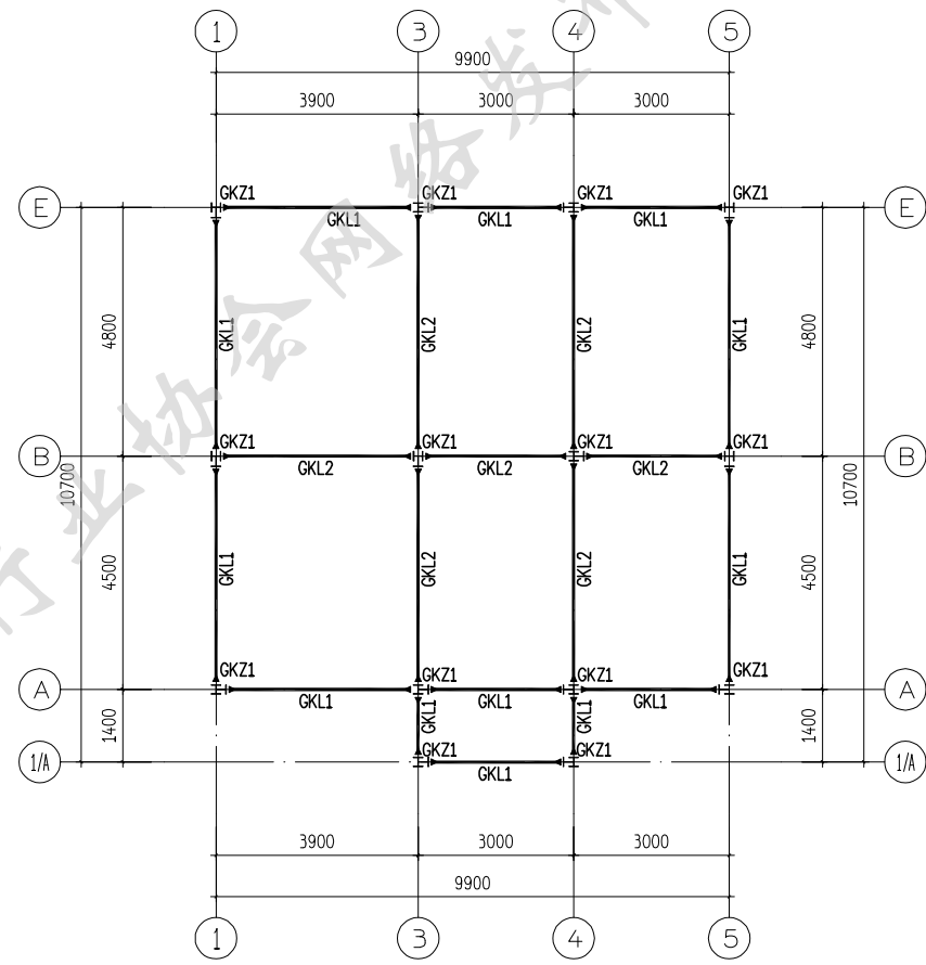
屋面结构平面布置图 6.130
