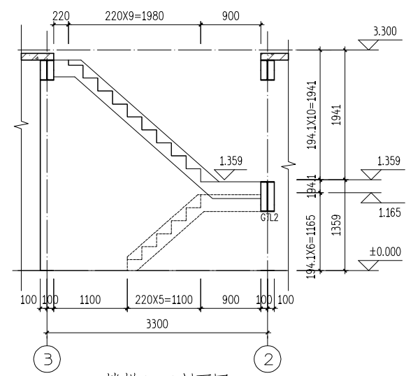
楼梯4-4剖面图
