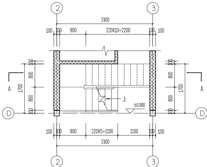
楼梯一层平面 1:50
