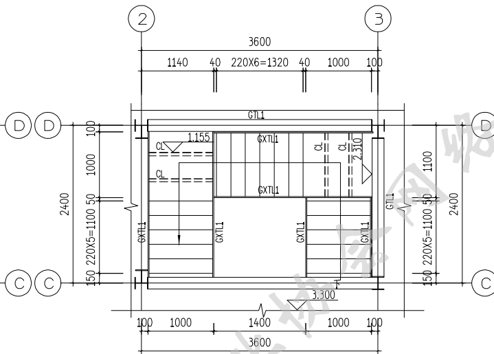
楼梯二层平面图 本楼梯适用于150平方米户型
