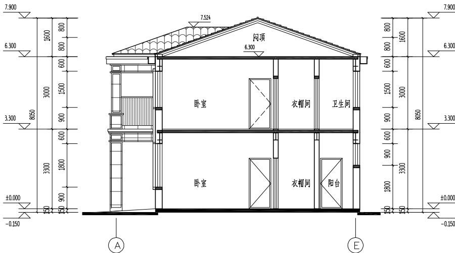
1-1剖面图 1:100
