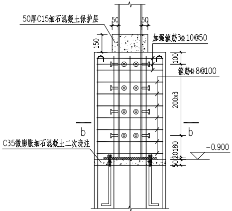
GKZ2柱脚节点详图
