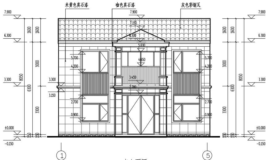
南立面图 1:100
