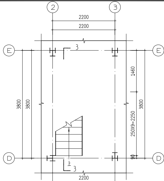
楼梯一层平面图
