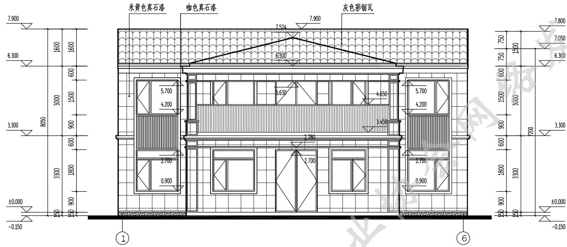
南立面图 1:100
