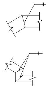
梯梁转角节点
