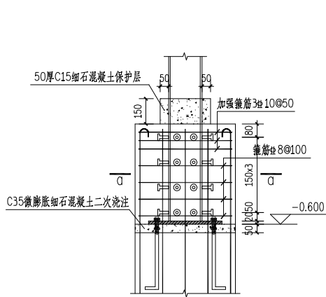
GKZ1柱脚节点详图
