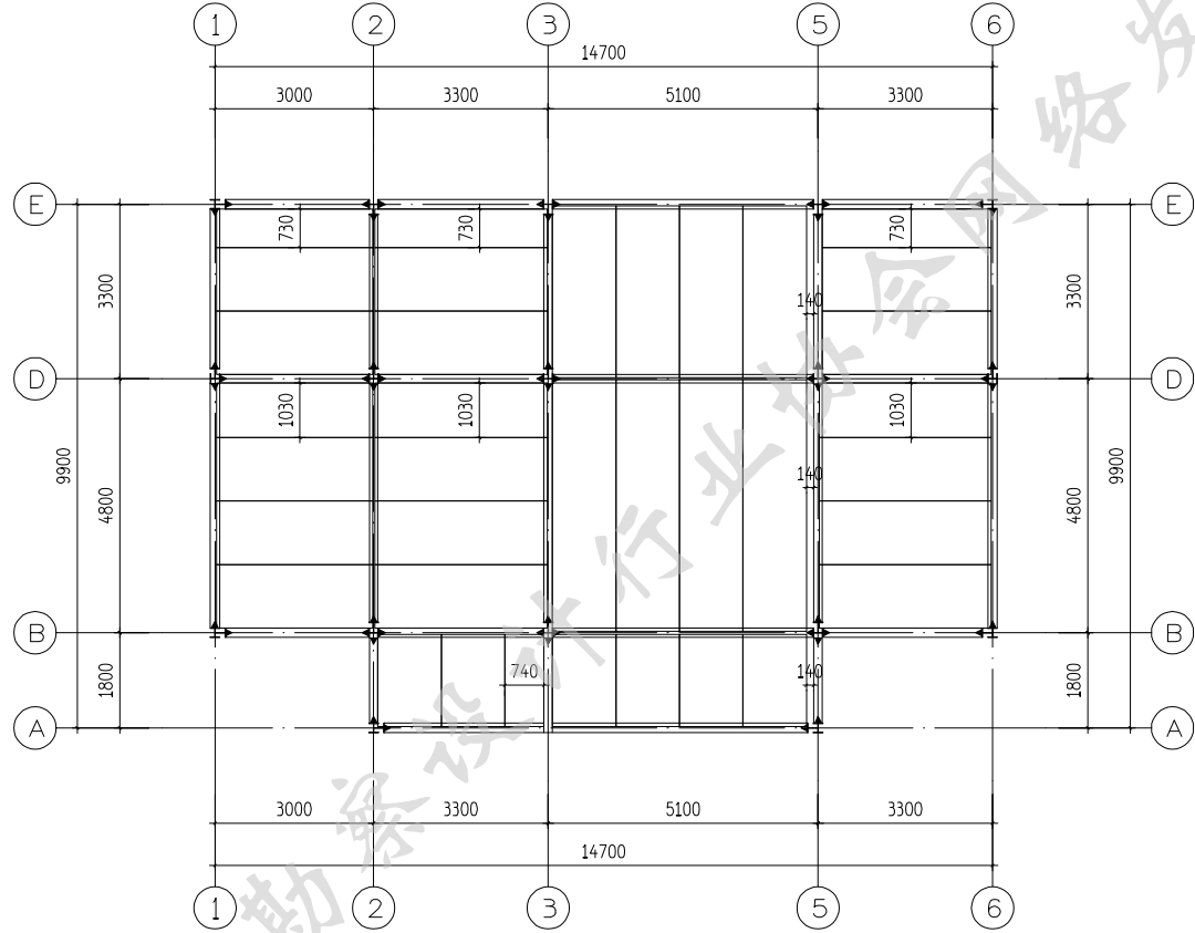
屋面SP板排布图 6.250
