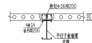
板侧与中间梁连接做法
