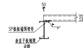
板与边梁搭接做法
