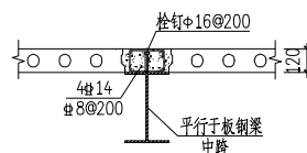
板侧与中间梁连接做法
