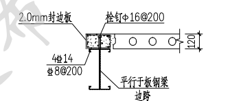
板侧与边梁连接做法
