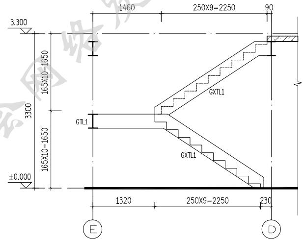
3-3剖面详图
