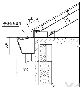
檐沟节点 1:20
