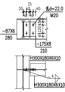
梁与梁铰接节点三
