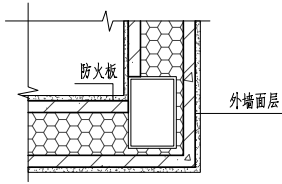
阳角节点 1:20
