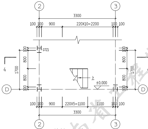
楼梯一层平面图
