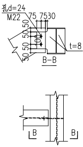
GXTL1与GTL1铰接
