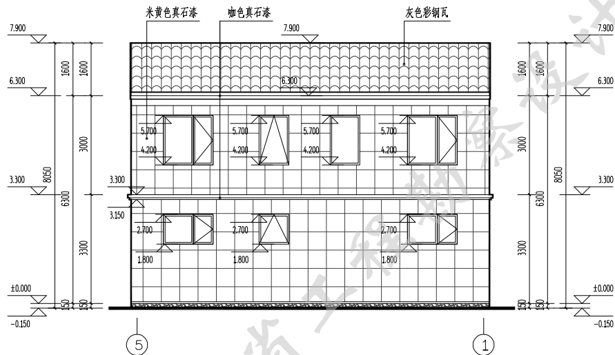
北立面图 1:100
