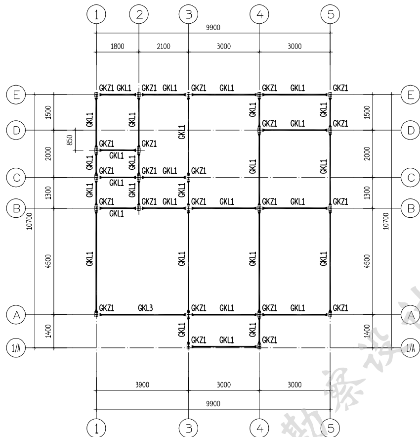
二層結構平面布置圖 3.130
