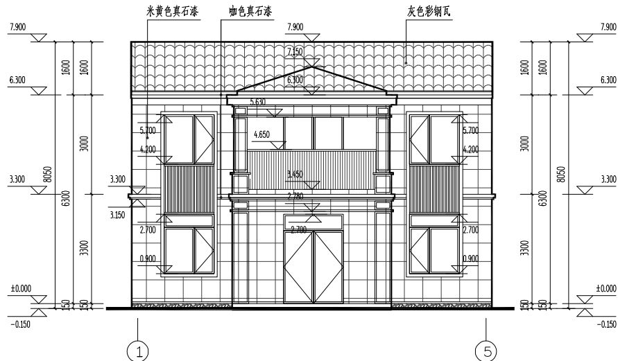
南立面图 1:100
