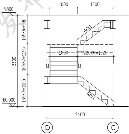
楼梯1-1剖面图 本楼梯适用于150平方米户型
