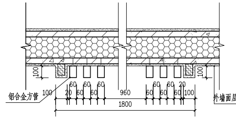
格栅造型节点 1:20
