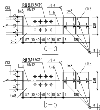
梁与柱刚接节点一
