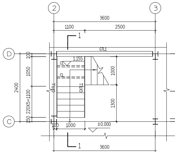
楼梯一层平面图 本楼梯适用于150平方米户型
