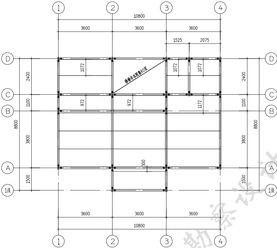
二层SP板排布图 3.250
