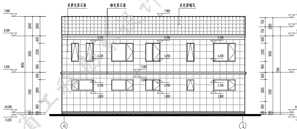
北立面图 1:100
