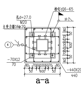
GKZ1柱脚节点详图
