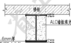
钢梁防火构造
