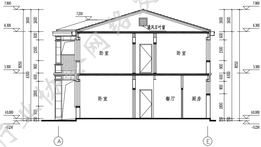
1-1剖面图 1:100
