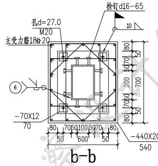
GKZ2柱脚节点详图
