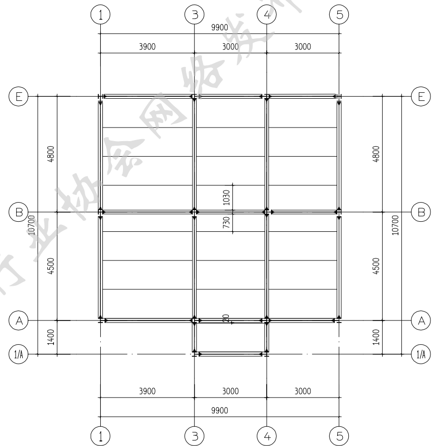
屋面SP板排布图 6.250
