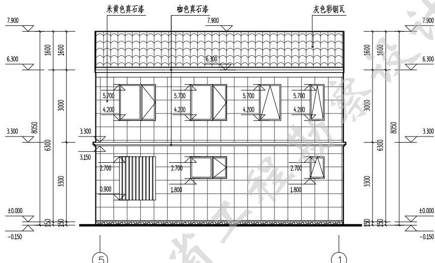
北立面图 1:100
