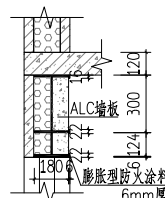
外墙窗顶钢梁防火构造
