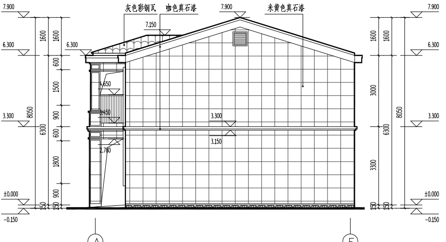
东立面图 1:100
