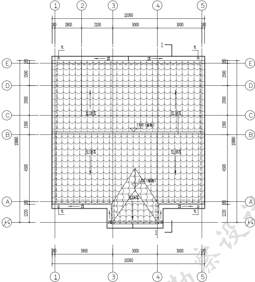
200平方米户型屋面平面图 1:100
