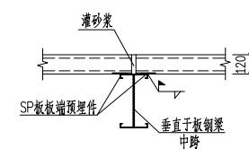
板与中间梁搭接做法
