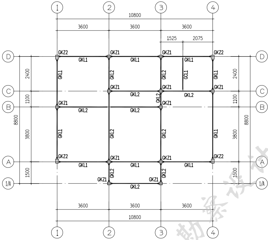
二层结构平面布置图 3.130
