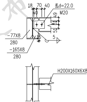
梁与梁铰接节点二
