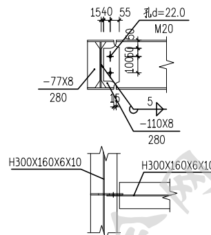
梁与梁铰接节点一
