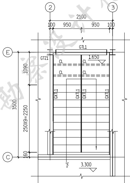
楼梯二层平面图 本楼梯适用于200平方米户型
