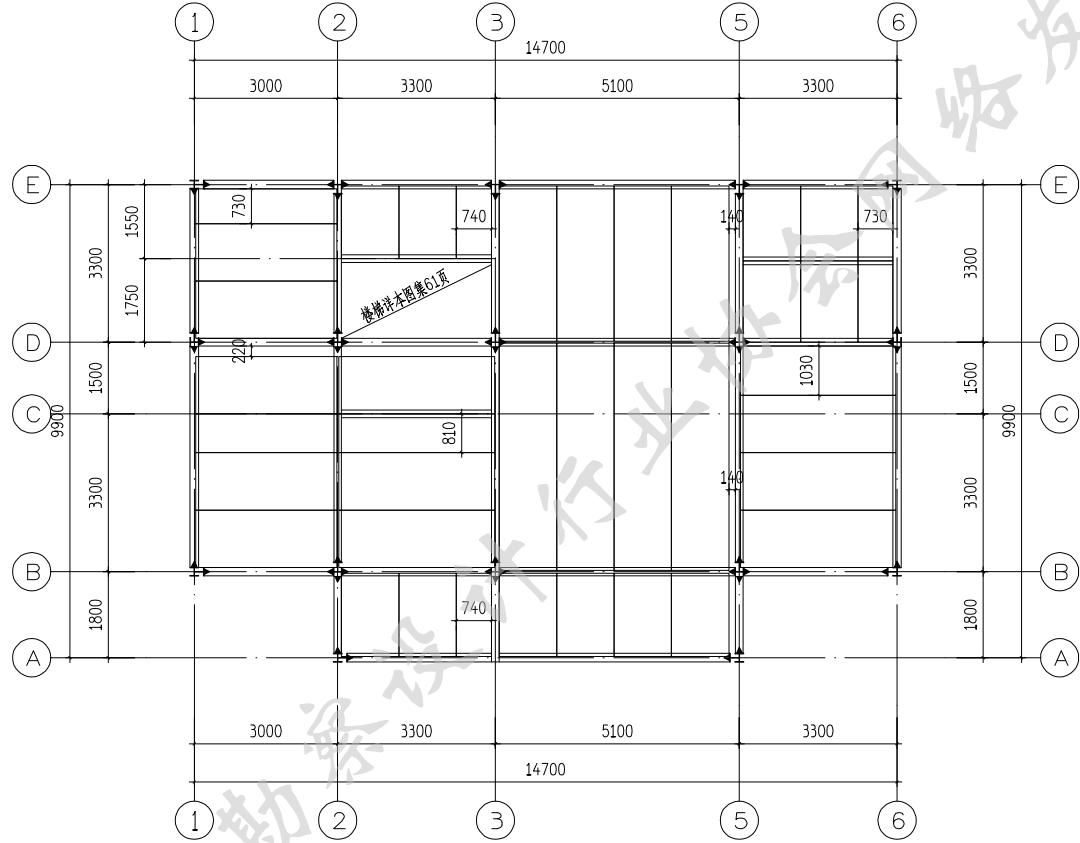
二层SP板排布图 3.250
