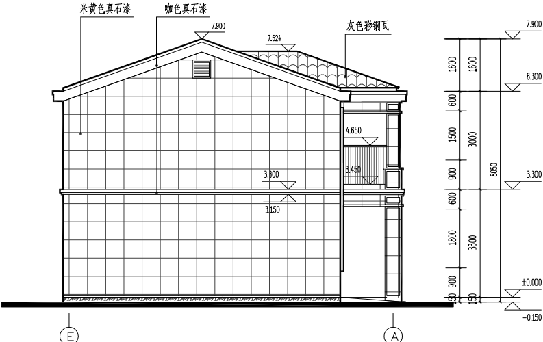
西立面图 1:100
