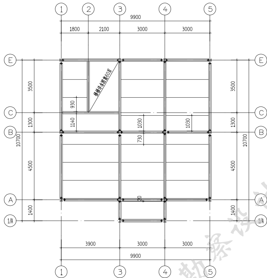
二層SP板排布图 3.250
