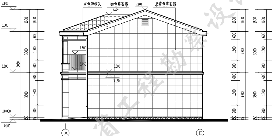
东立面图 1:100
