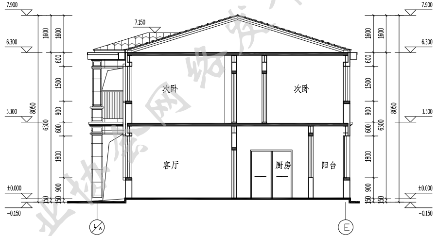
1-1剖面图 1:100
