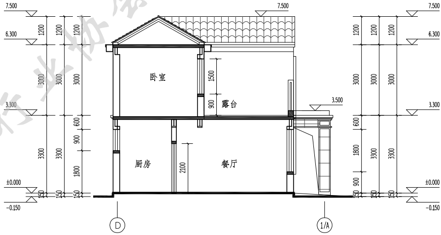
1-1剖面图 1:100
