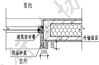
窗侧口节点 1:20
