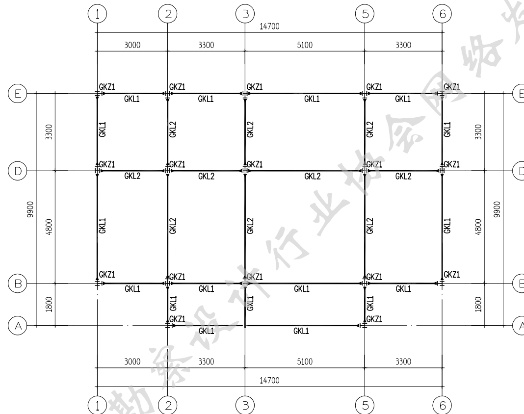
屋面结构平面布置图
