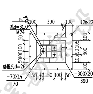
板侧与中间梁连接做法
