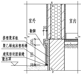
勒脚节点 1:20
