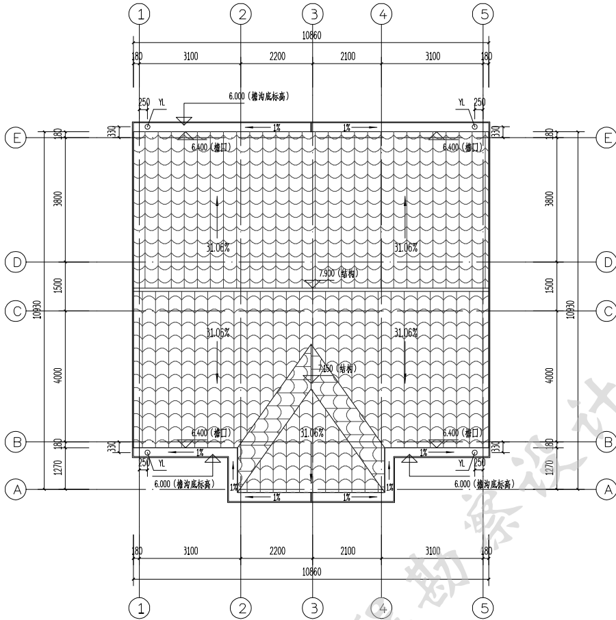
220平方米户型屋顶平面图 1:100
