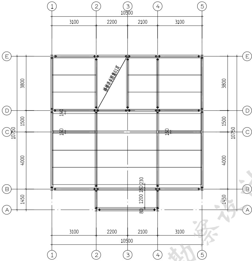
二层SP板排布图 3.250
