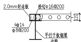
板侧与边梁连接做法
