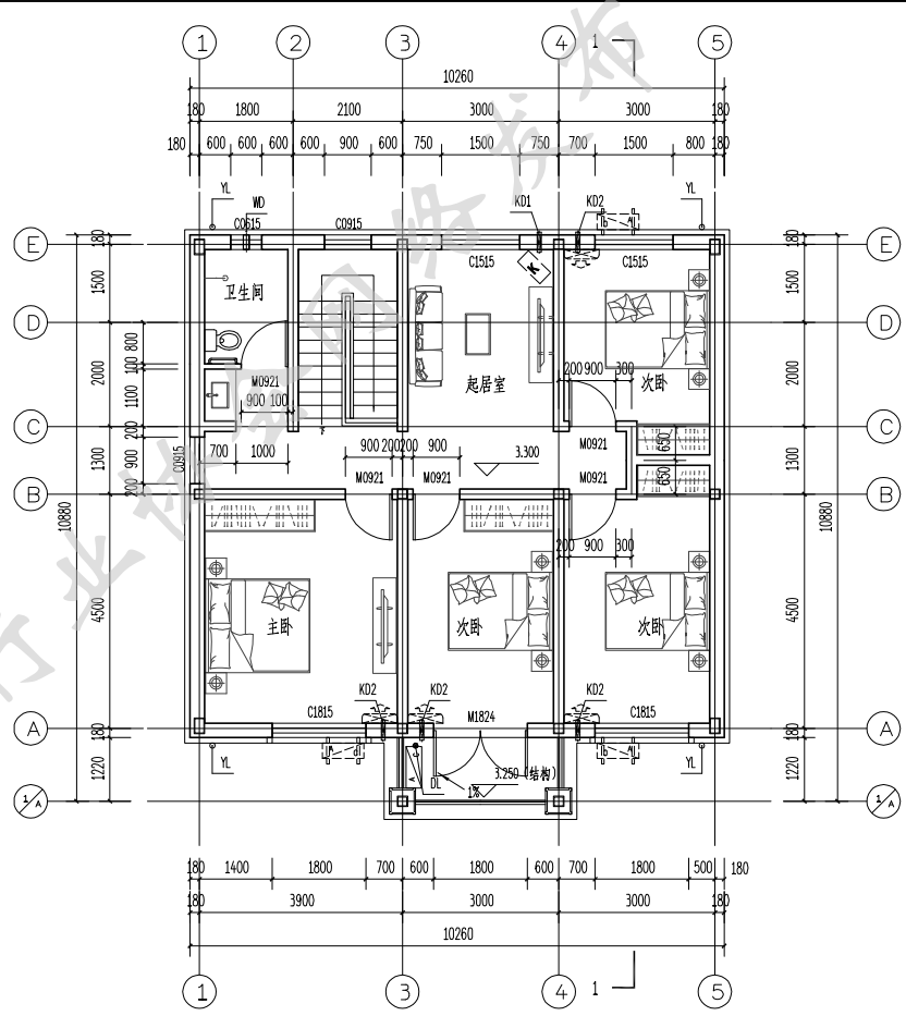
200平方米户型二层平面图 1:100
