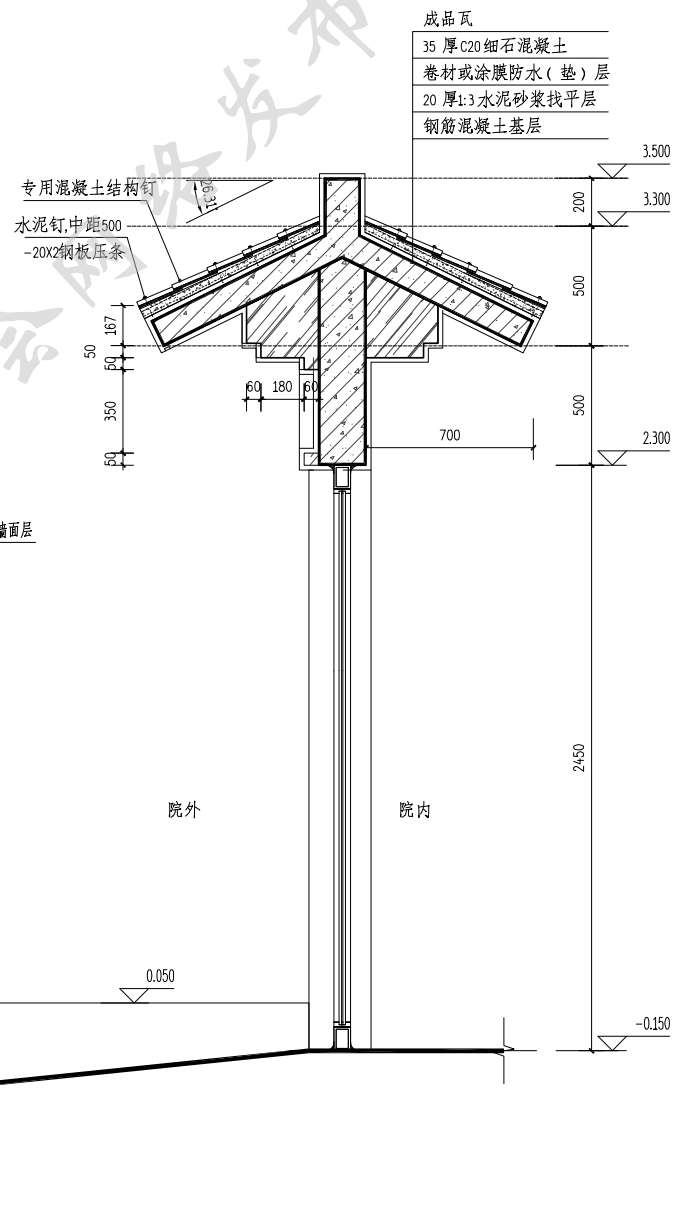
围墙a-a剖面图 1:20
