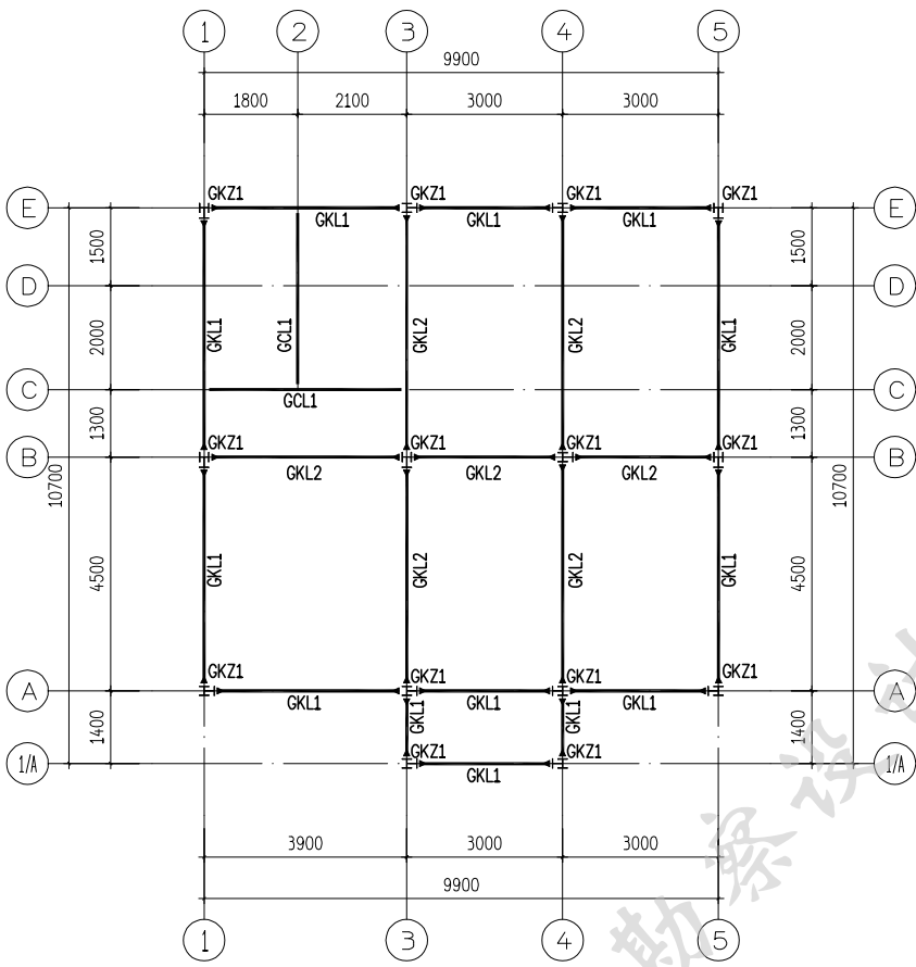
200平方米户型结构平面布置图 3.130
