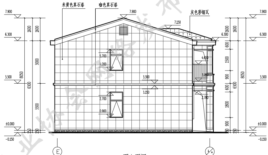
西立面图 1:100
