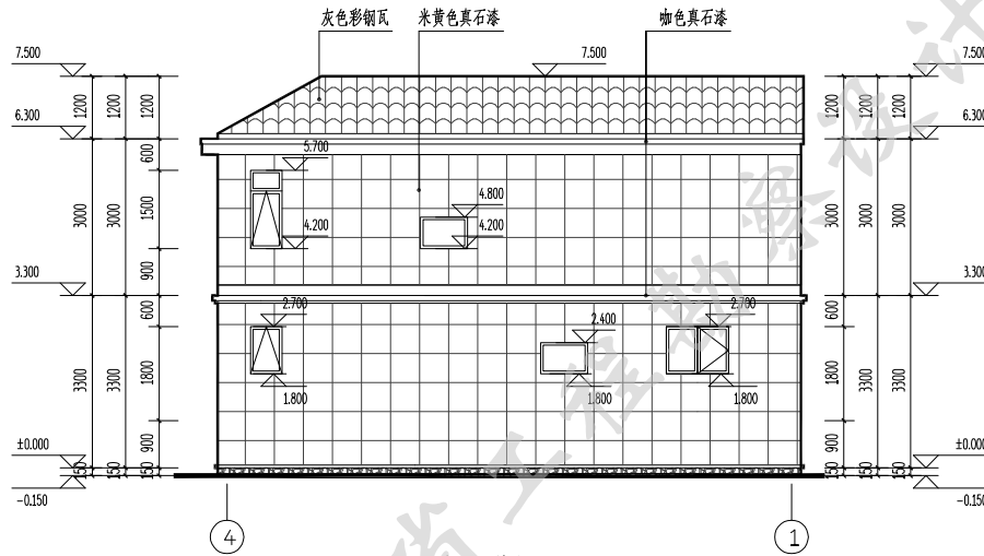
北立面图 1:100
