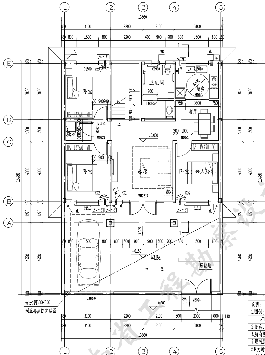
220平方米户型一层平面图 1:100
