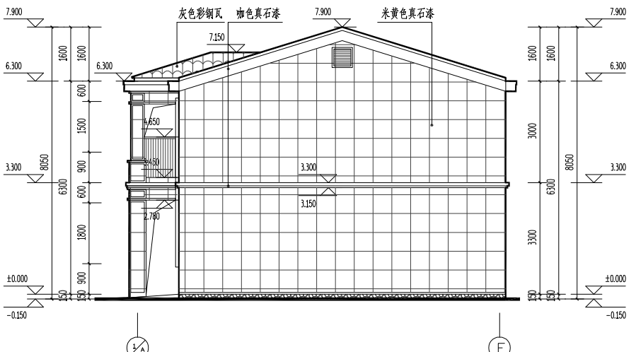
东立面图 1:100
