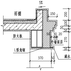
雨棚节点 1:20
