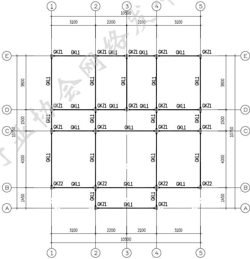
屋面結構平面布置圖 6.130
