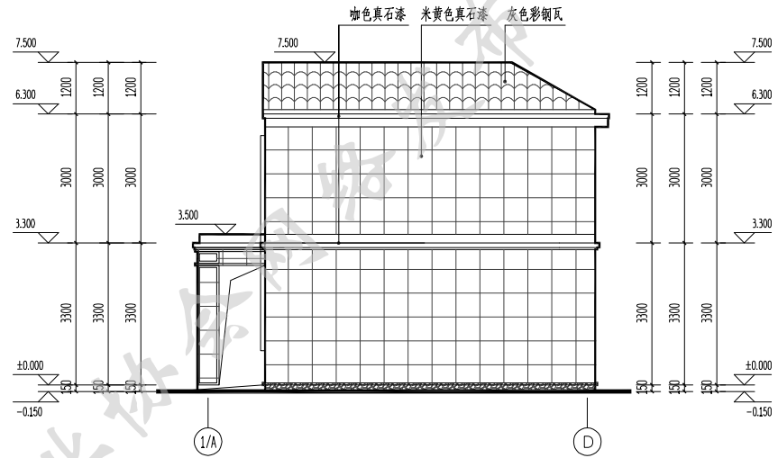
东立面图 1:100
