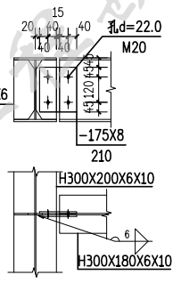
梁与梁铰接节点二
