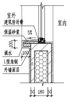
外窗下口节点 1:20
