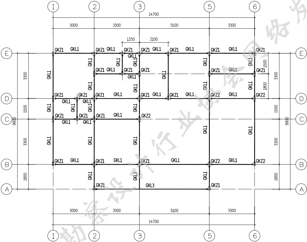
二层结构平面布置图 3.130
