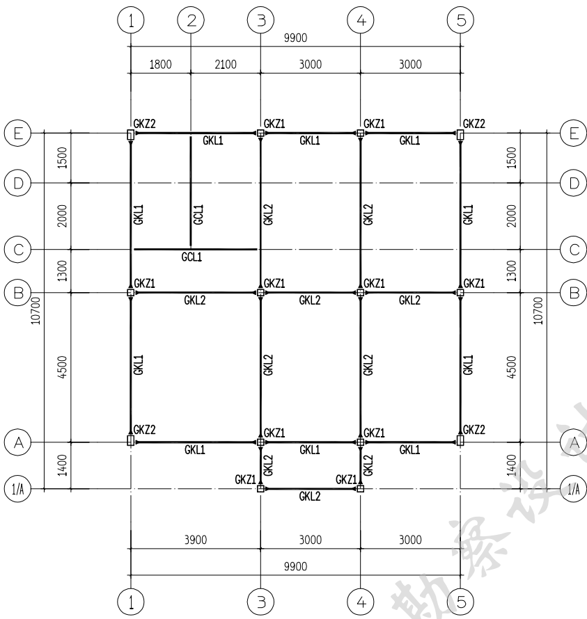
二层结构平面布置图 3.130
